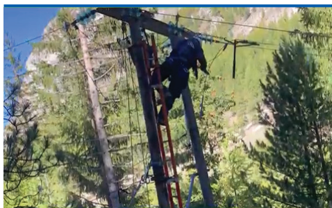
Chantier de réparation d'un tronçon aérien HTA sur le site de BRAMANS
