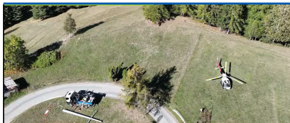
Photo aérienne de la réparation d'un tronçon aérien HTA à BRAMANS
